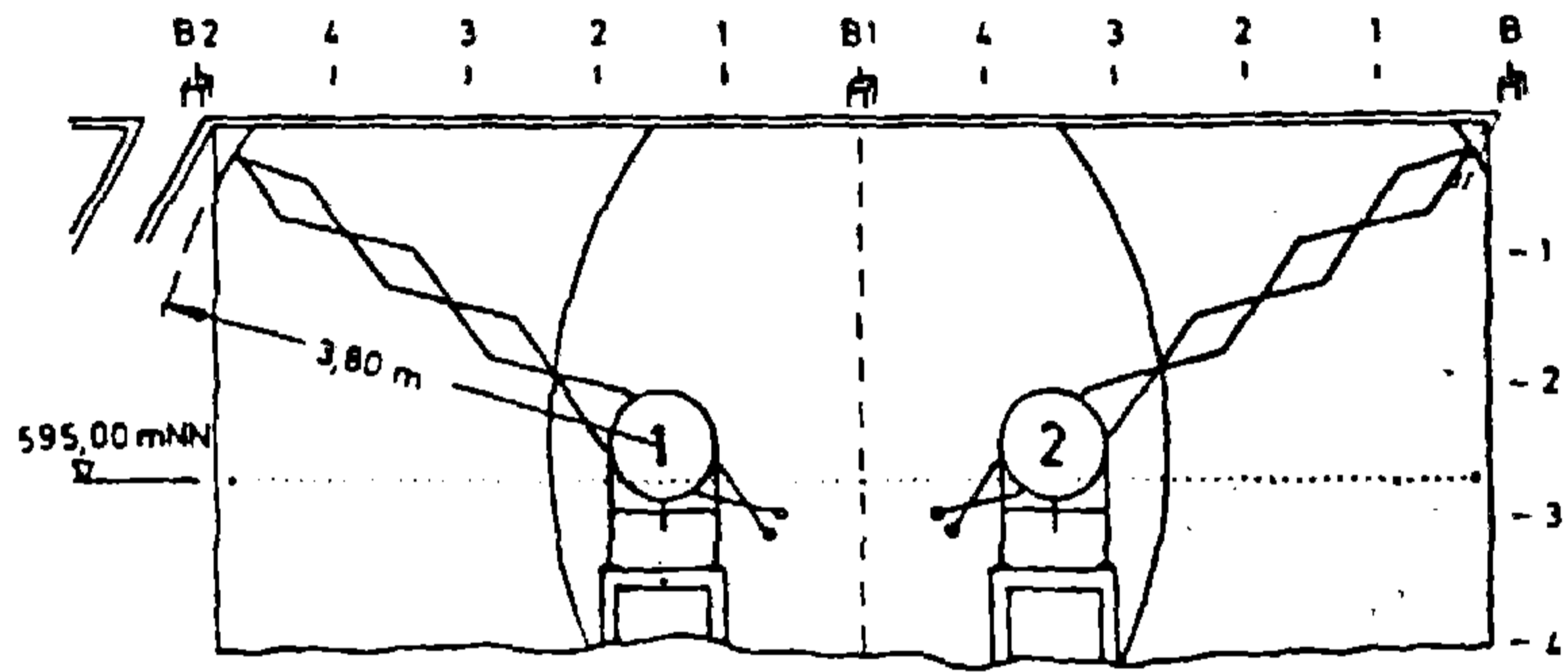
(شكل ٢٥) نقط الارتكاز في الموقع
